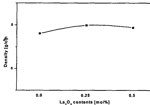
그림 1. \text{La}_2\text{O}_3 첨가량에 따른 밀도변화.
