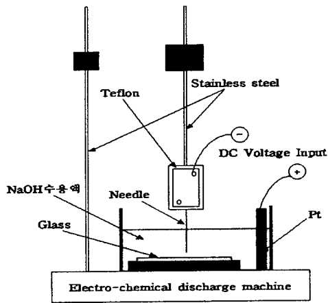
그림 1. 전해방전가공기의 구조 Fig. 1. Structure of electro-chemical discharge machine
