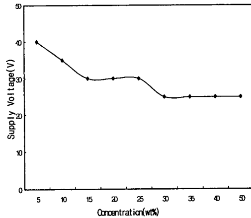
그림 3. 농도에 대한 미세 구멍 생성 전압 Fig. 3. Hole creating voltage as a function of NaOH concentration
