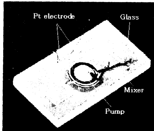
그림 6. 유체분석소자 Fig. 6. Liquid analyzer
