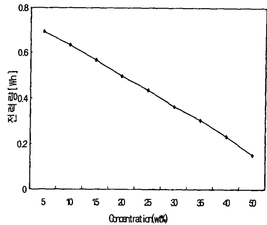
그림 5. 농도에 대한 전력량 Fig. 5. Electric power as a function of NaOH concentration
