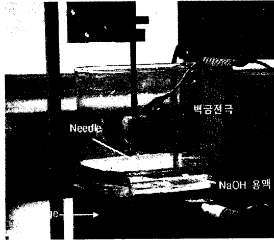
그림 2. 전해방전가공기의 사진 Fig. 2. Photograph of the electro-chemical discharge machine
