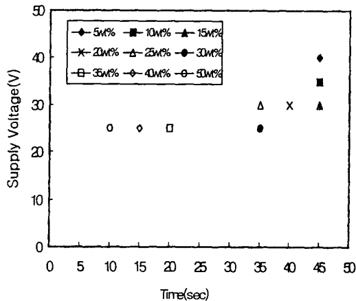
그림 4. 미세 구멍 생성 시점 Fig. 4. Hole creating time
