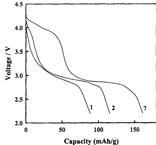
그림 5. \text{LiMnO}_2/\text{Li} 전극의 방전 곡선.
