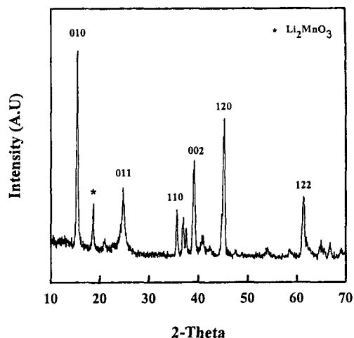
그림1. \text{LiMnO}_2 의 X-선 패턴.
