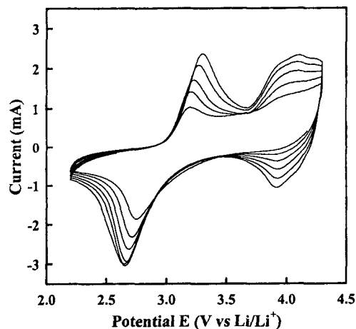
그림 2. \text{LiMnO}_2/\text{Li} 전극의 순환전압전류특성.
