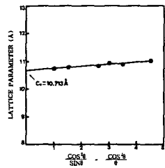
그림 5. CdGa₂Se₄의 격자 상수 c₀ Fig. 5. Lattice parameter c₀ of CdGa₂Se₄
