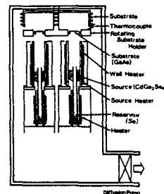
그림 2. HWE 장치의 개략도
