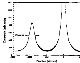
그림 7. CdGa₂Se₄ 단결정 박막의 이중 결정 X-선 요동곡선 Fig. 7. Double crystal X-ray rocking curve of CdGa₂Se₄ single crystal thin film.
