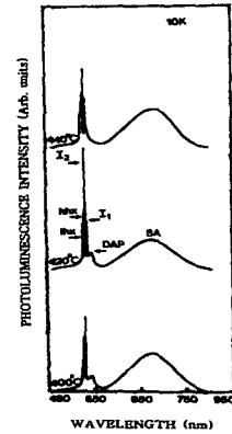
그림 6. CdGa₂Se₄ 단결정 박막의 기판 온도 변화에 대한 10K에서 PL 스펙트럼 Fig. 6. PL spectrum at 10K according to the substrate temperature variation.
