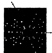
그림 8. 배면 반사법으로 측정된 (112)면의 Laue 무늬 Fig. 8. Black-reflection Laue patterns for the (112) planes.
