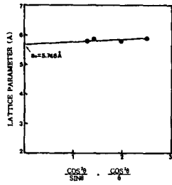
그림 4. CdGa₂Se₄의 격자 상수 a₀ Fig. 4. Lattice parameter a₀ of CdGa₂Se₄
