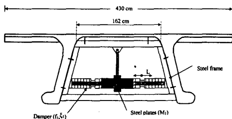
그림 14. Horizontal TMD
