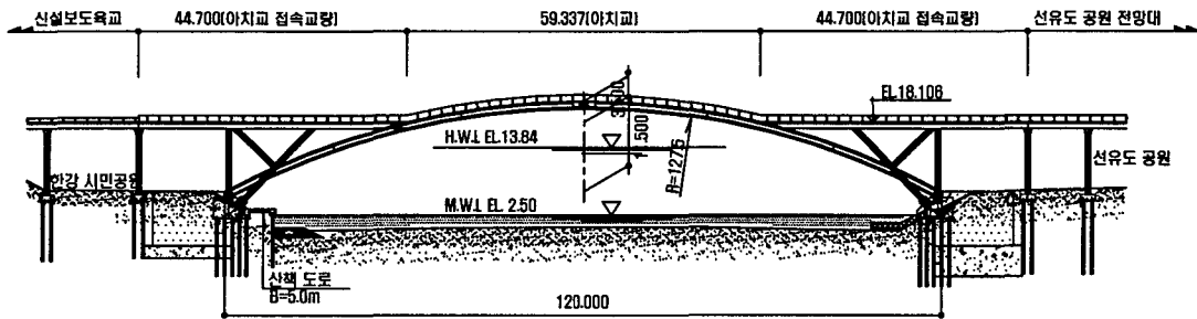
그림 6. 아치교 계획현황
