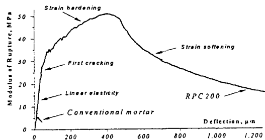
그림 2. RPC의 휨강도 특성
