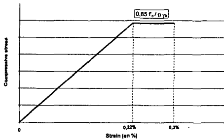
그림 9. 압축강도곡선
