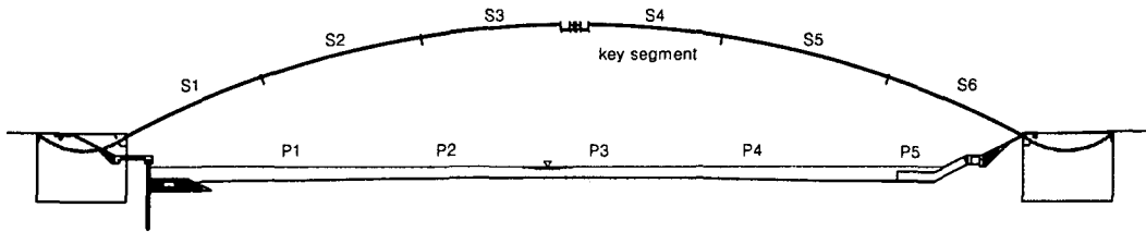
그림 18. 아치교 가설개요도
