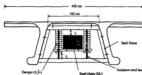
그림 15. Vertical TMD
