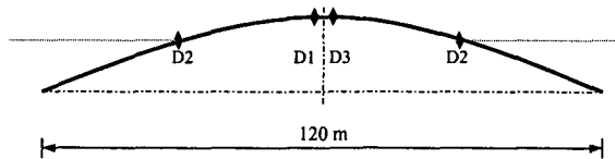
그림 13. TMD 설치위치
