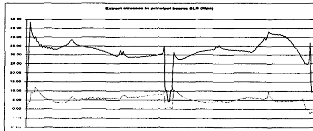
그림 11. 부재위치별 최대, 최소 발생응력
