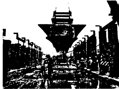
그림 17. Segment의 이동전경
