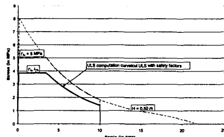
그림 10. 인장강도곡선
