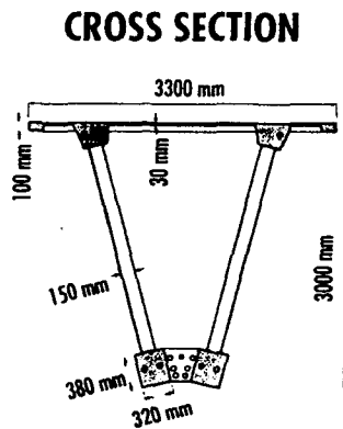
그림 4. 횡단면의 구성
