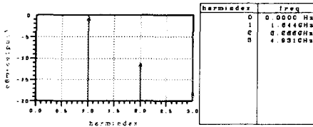
(그림 7) PCS 출력주파수 Fig. 7 PCS output frequency
