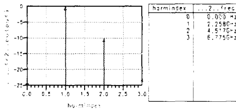
(그림 3) IMT2000 출력 발진주파수 Fig. 3 IMT2000 output frequency
