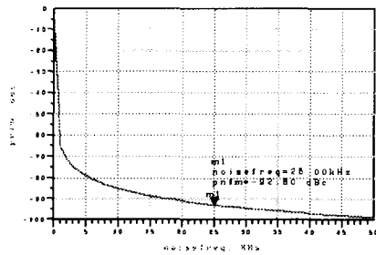
(그림 8) PCS 위상잡음 Fig. 8 PCS phase noise
