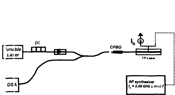
그림 1. 다파장 스위칭과 파장 변환 실험을 위한 실험 구성도
