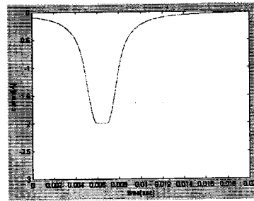
그림. 2 브러시리스 직류 전동기의 전류 응답 Fig.2 Current Response of Brushless DC Motor
