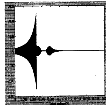
그림. 4 브러시리스 직류 전동기의 제어입력 Fig.4 Control input of Brushless DC Motor
