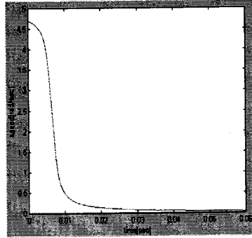
그림. 1 브러시리스 직류 전동기의 속도 응답 Fig.1 Speed Response of Brushless DC Motor
