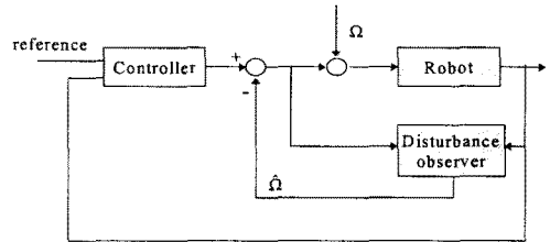
그림 1. 외란관측기 구조 Fig 1. Disturbance observer
