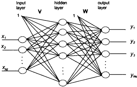
그림 2. 다층 신경망 제어기 Fig. 2 MLP network
