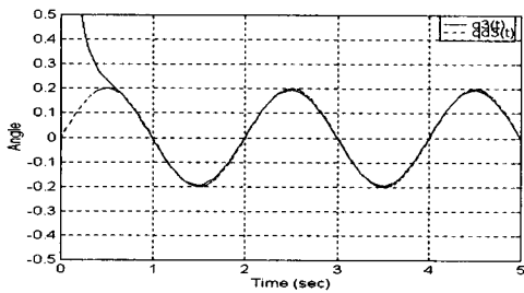
그림 4. 제어결과 Fig. 4. Control result
