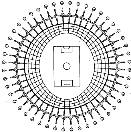
그림 2. 케이블지붕의 평면
