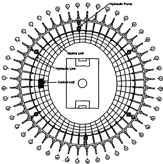
그림 3. 리프팅시스템의 배치
