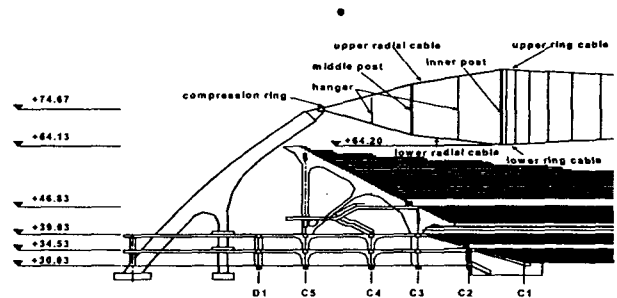
그림 1. 케이블지붕의 구성
