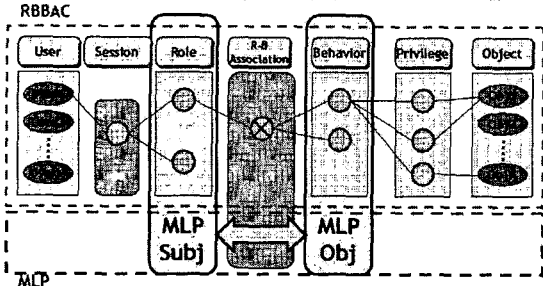
[그림 1] ML-RBBAC 모델의 개념도
