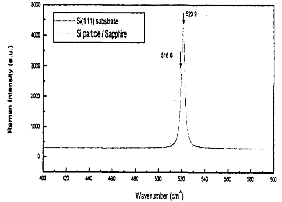
그림 5. 수소 처리된 Si 기판과 사파이어 기판 위의 원추형 Si particle의 라만 스펙트럼
