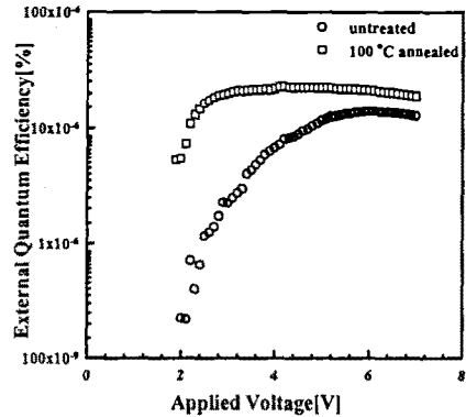
그림 4. 100°C 열처리한 소자와 비열처리소자의 외부양자 효율.
