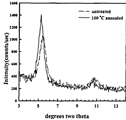
그림 2. 비열처리와 100°C 열처리 P3HT막의 XRD. Fig. 2 X-ray diffraction pattern of untreated and 100°C annealed P3HT films.
