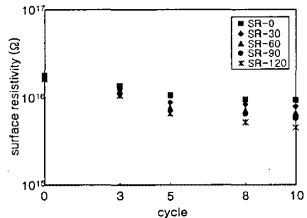
그림2. 반복열화에 따른 표면저항률의 변화
