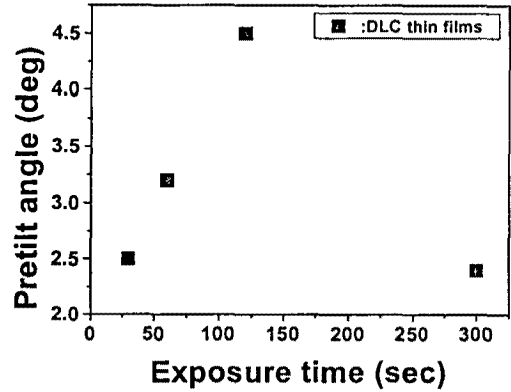
그림 5. DLC 박막 표면에 IB 조사시의 조사시간에 따른 네마틱 액정의 프리틸트각의 발생. Fig. 5. Generation of pretilt angle in NLC by IB exposure on the DLC thin film surfaces as a function of exposure time.
