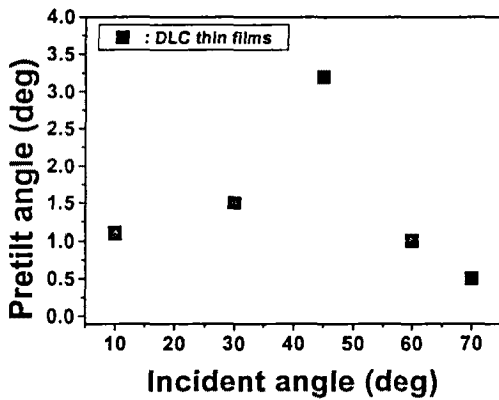
그림 4. DLC 박막 표면에 편광된 IB을 1분간 조사시의 입사각도에 따른 네마틱액정의 프리틸트각의 발생. Fig. 4. Generation of pretilt angles in NLC with IB exposure on the DLC thin film surfaces for 1 min as a function of incident angle.
