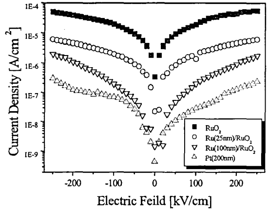
그림 3. 하부전극에 따른 PZT 박막의 I-V 특성 Fig. 3. I-V characteristics of PZT thin films as a bottom electrode
