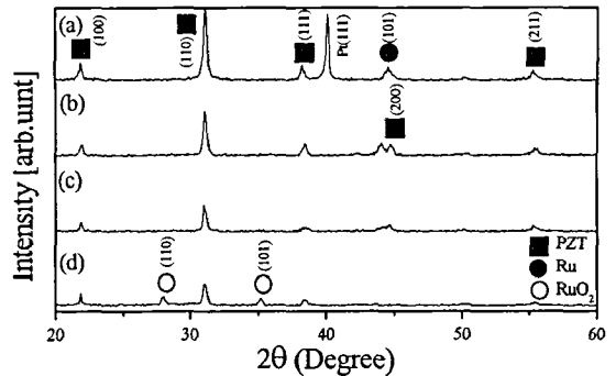
그림 1. 하부전극에 따른 PZT 박막의 XRD 패턴 (a) Pt, (b) Ru(100nm)/RuO 2 , (c) Ru(25nm)/RuO 2 , (d) RuO 2
