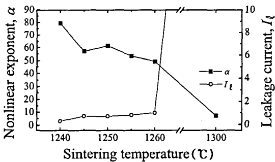
그림 4. 소결온도에 따른 ZnO-Pr 6 O 11 -CoO-Cr 2 O 3 -La 2 O 3 계 바리스터의 비직선 지수와 누설 전류.
