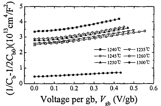
그림 5. 소결온도에 따른 ZnO-Pr 6 O 11 -CoO-Cr 2 O 3 -La 2 O 3 계 바리스터의 (1/C_b-1/2C_{bo})^2 vs. V_{gb} .
