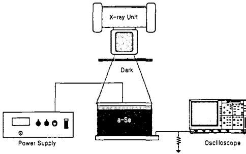
Fig 3. X-ray sensitivity 측정을 위한 시스템 구성도
