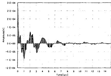
그림 1. 임펄스 응답의 Pulse model 적용
