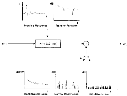
그림 9. 전력선 채널 모델
