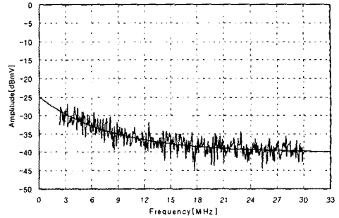
그림 5 배경 잡음 모델
