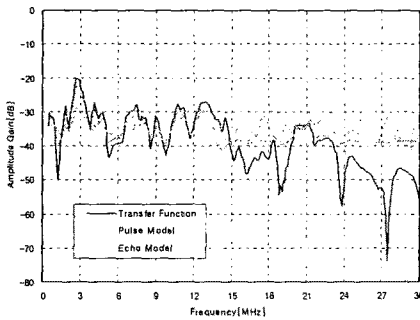
그림 3. 전달함수의 실측치 및 모델링 구현 결과
