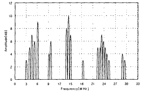
그림 6 협대역 잡음 모델
