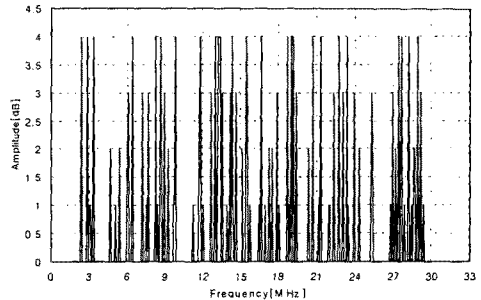
그림 7 충격 잡음 모델
