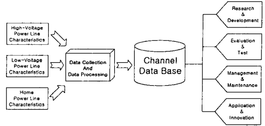
그림 10. 채널 Data Base 구성
