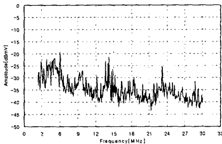
그림 4. 전력선 채널 실측 잡음
