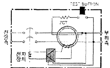
[ 그림 2 : 누전차단기의 구성도 ]
