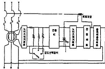
[ 그림 1 : 전자회로 구성도 ]
