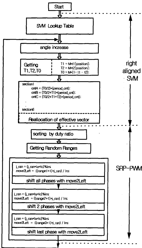
그림5 2상 및 3상 SRP-PWM의 구현 Fig.5 Implementation of two-phase and three-phase SRP-PWM
