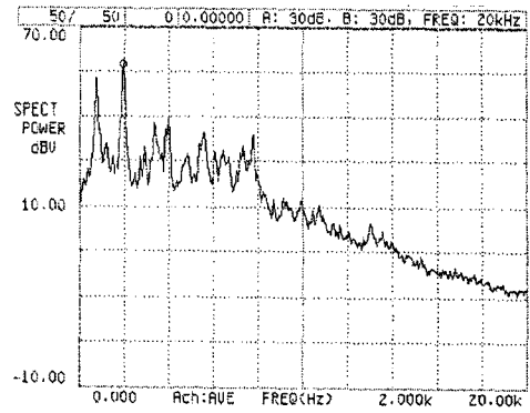
(d) 2 phase SRP-PWM
