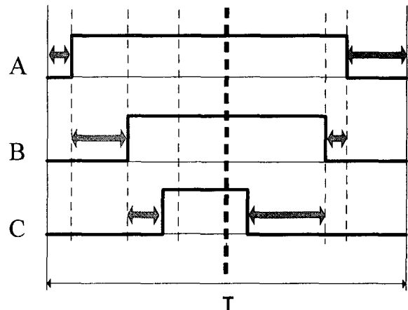
그림2 3상 SRP-PWM 각상의 펄스 Fig.2 Each phase pulse with three-phase SRP-PWM
