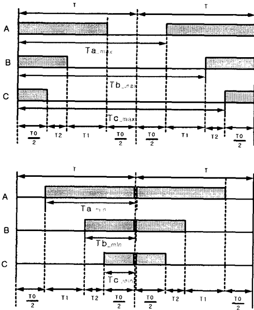
그림4 최대 및 최소 유효 스위칭 주파수 Fig.4 Maximum and minimum effective switching frequency
