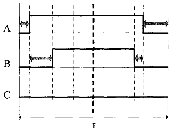
그림3 2상 SRP-PWM 각상의 펄스 Fig.3 Each phase pulse with two-phase SRP-PWM
