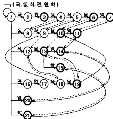
그림 1. DER 구조의 goto, failure와 reverse 함수
