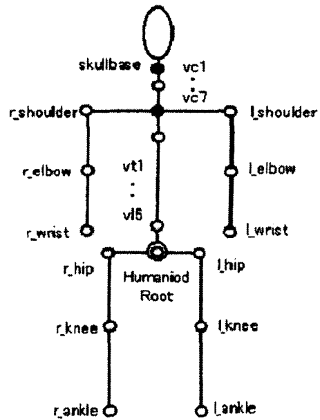
그림 2. X3D Humanoid joint node
