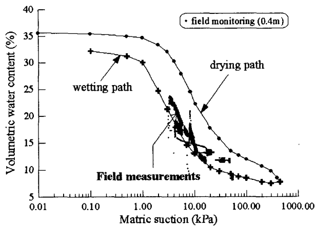
그림 6. 0.4m 깊이에서의 현장 흡-수분 특성
