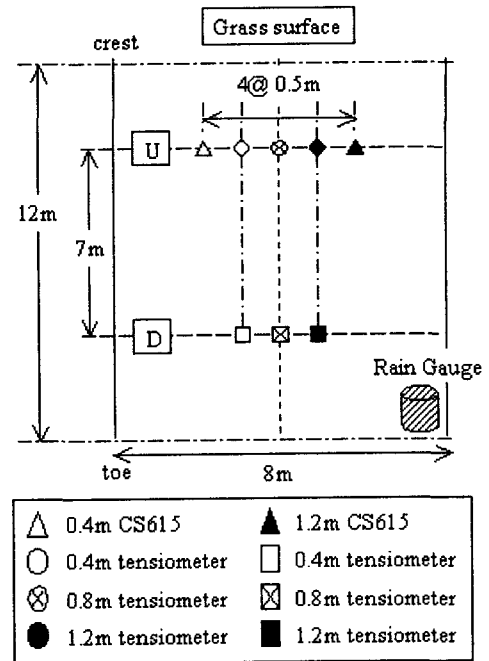
그림 2. 계측장비 배치도
