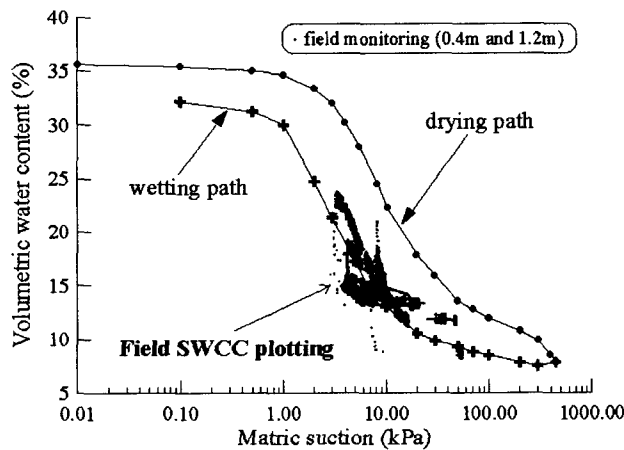
그림 8. 대상 지반의 현장 흡-수분 특성
