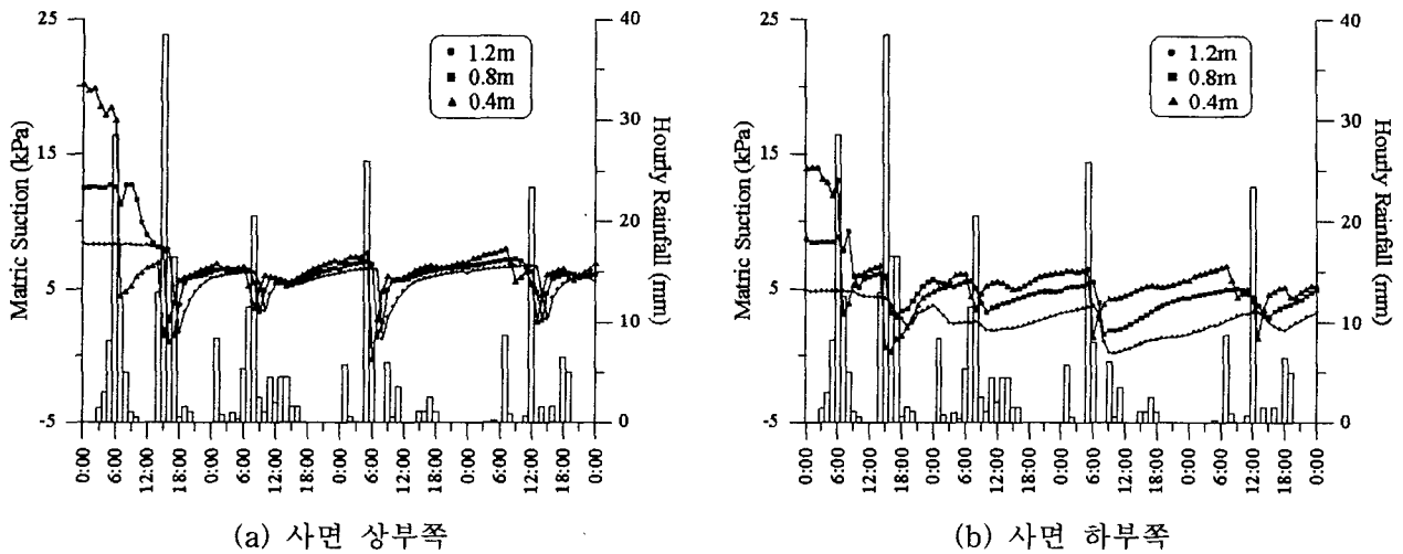
그림 5. 모관흡수력의 시간별 변화양상(7월29일~8월1일)
