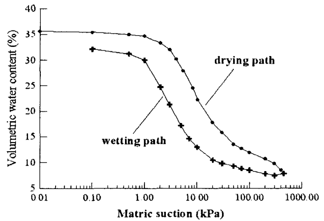
그림 1. 흡-수분 특성곡선
