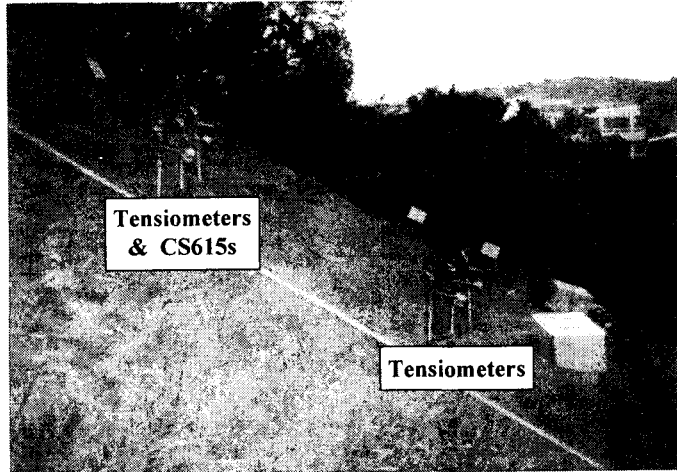
사진 1. 계측장비가 설치된 현장 사면
