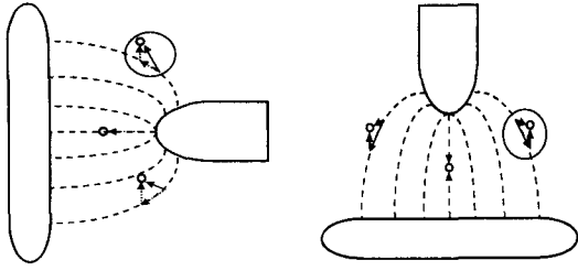
(a)기포거동 개념도(I) (b)기포거동 개념도(II)
