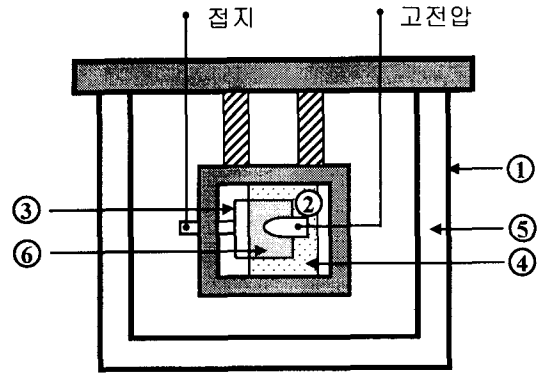
① Pyrex glass ② Knife type 전극 ③ 평판 전극 ④ 전극 지지판 ⑤ 진공 ⑥ 고체 절연재료
