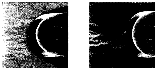
(a) DC(+), 10[mm] (b) DC(-), 10[mm]
