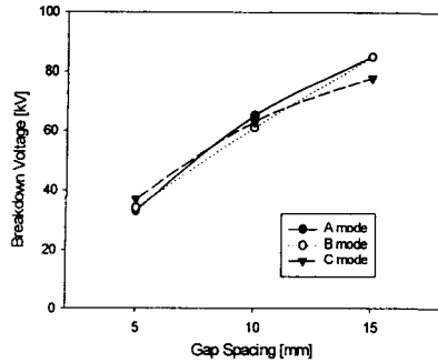
(b) 부극성 연면방전 전압
