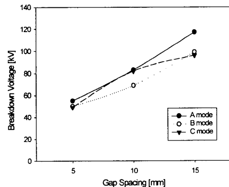
(a) 정극성 연면방전전압
