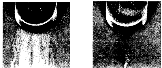
(a) DC(+), 10[mm] (b) DC(-), 10[mm]
