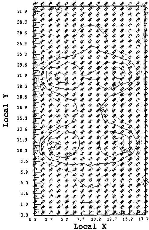
그림 11. 바닥면의 등조도 곡선
