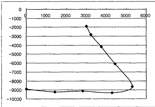
그림 2. v=90 에서의 목표 배광
