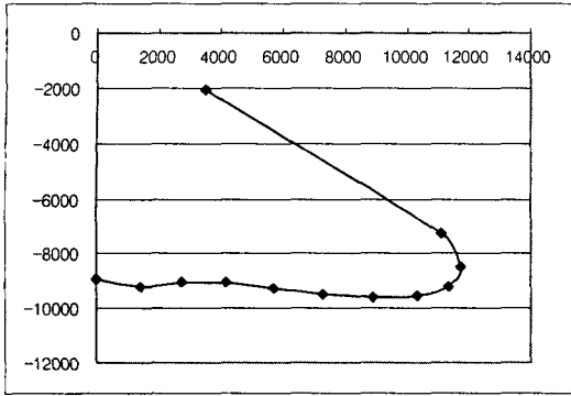
그림 1. v=0 에서의 목표 배광
