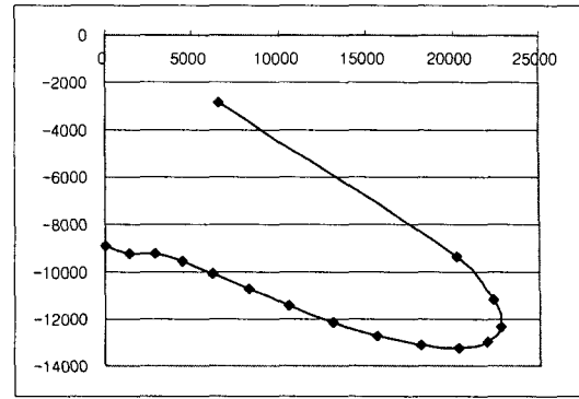
그림 4. v=270 에서의 목표 배광
