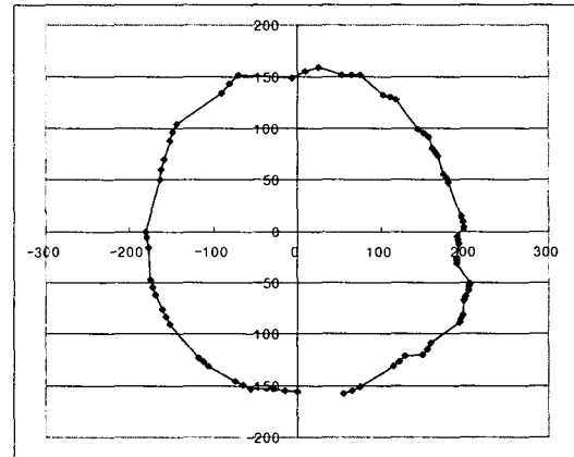
그림 5. \gamma, \delta 로 계산되어진 반사판 개구부 모양
