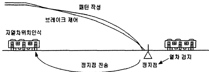
그림 1. D-ATC의 기본원리
