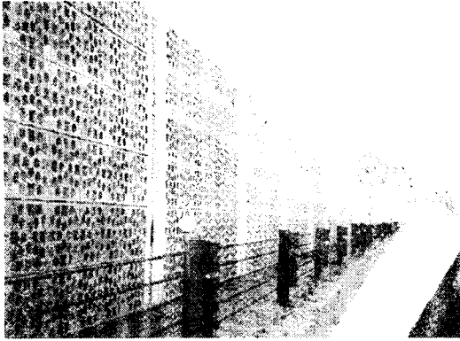
사진 3. 고속도로에 포러스콘크리트를 이용한 흡음판
