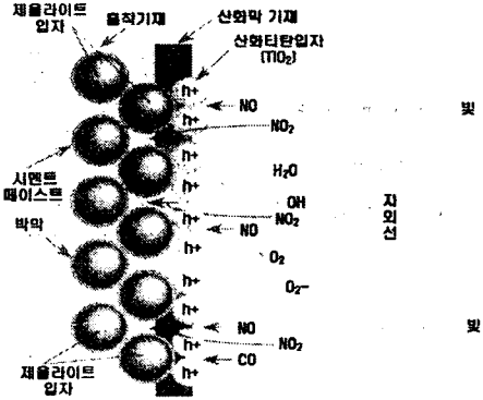
그림 3. 광촉매 TiO 2 와 제올라이트를 사용한 포러스콘크리트의 NO x 흡착 모식도
