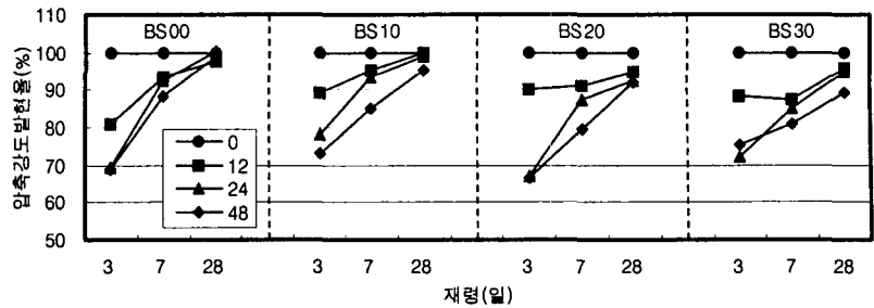
그림 3 재령별 압축강도 발현율(%, -10^{\circ}\text{C} , 동해시점 24시간후)
