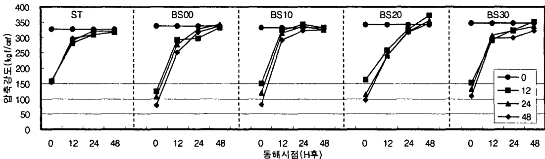
그림 2 동해시점에 따른 동해지속시간별 압축강도( -10^{\circ}\text{C} )
