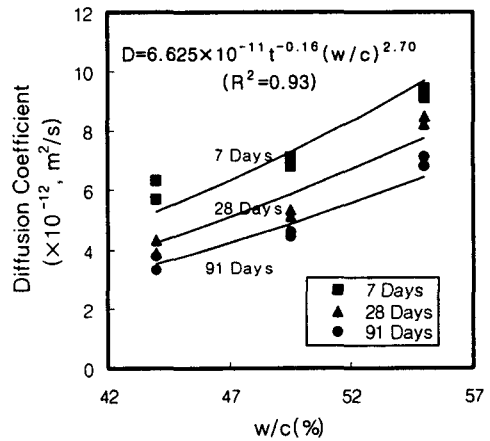
그림 4. 확산계수와 물-시멘트비 및 재령의 관계
