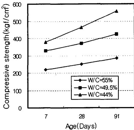
그림 1. 콘크리트의 압축강도
