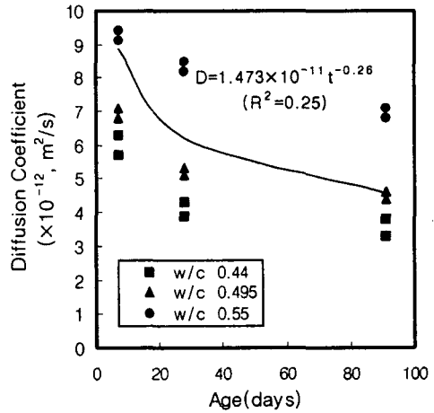
그림 2. 확산계수와 재령의 관계
