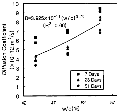
그림 3. 확산계수와 물-시멘트의 관계
