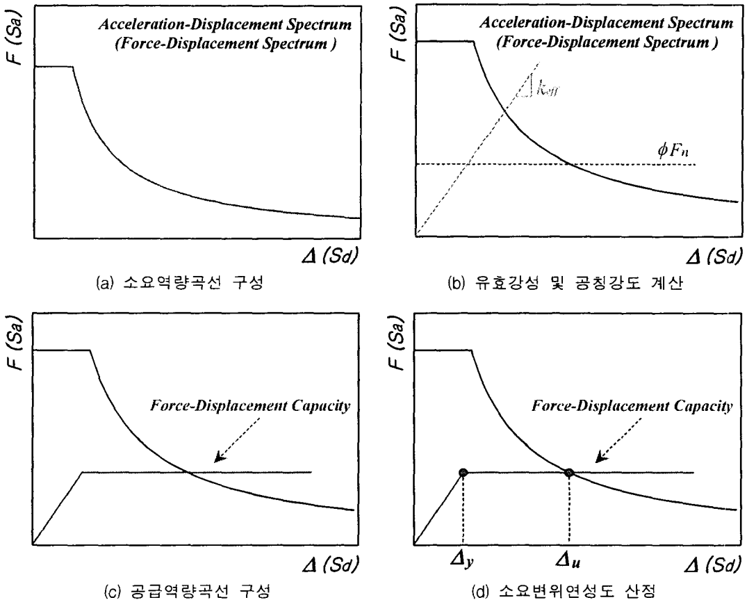
그림 2 연성도를 고려한 철근콘크리트 교각의 내진설계방법 과정
