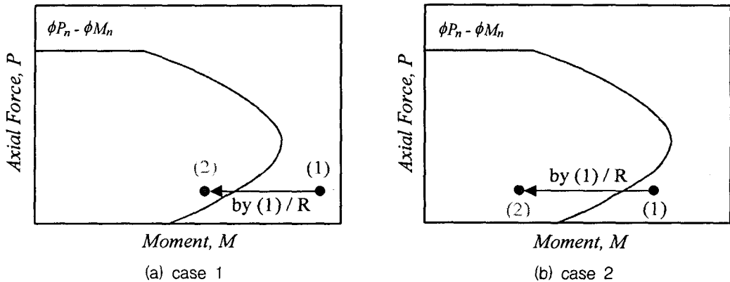
그림 1 응답수정계수를 적용한 철근콘크리트 교각의 내진설계 개념
