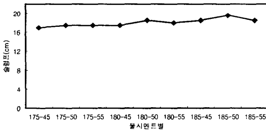
그림 1 단위수량과 물시멘트비별 슬럼프
