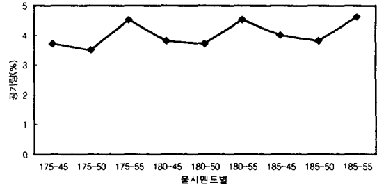
그림 2 단위수량과 물시멘트비별 공기량
