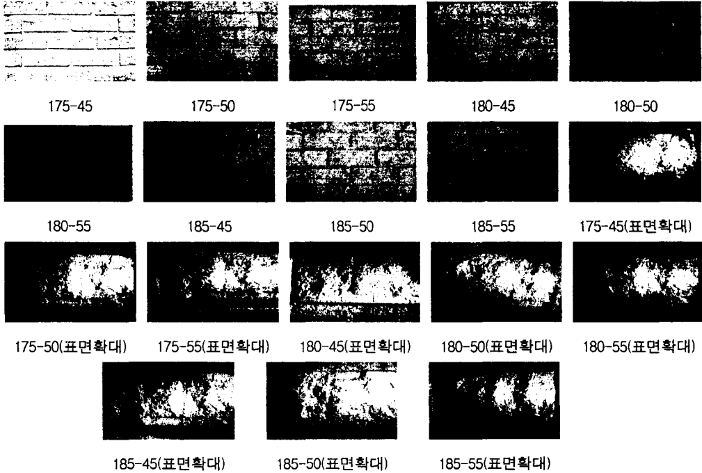
사진 1 단위수량과 물시멘트비 표면 사진
