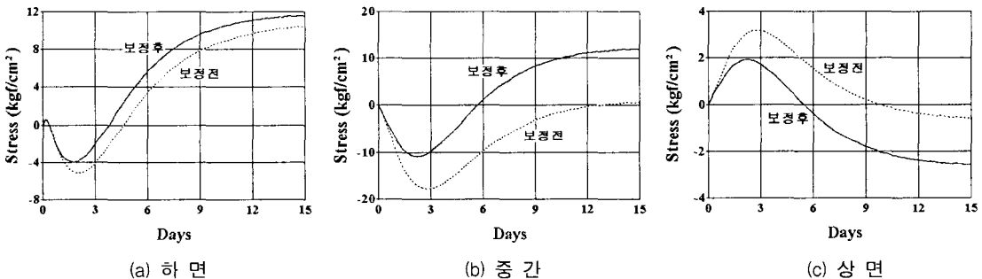
그림 2 ABAQUS로 해석한 수화열응력 (*ELASTIC을 사용한 재료모델)
