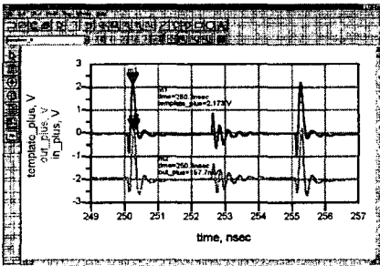
그림 12 (+) 펄스 복조기의 입출력 파형
