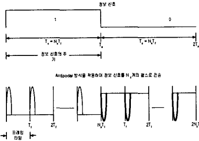
그림 2 Antipodal 방식에서 펄스의 구성
