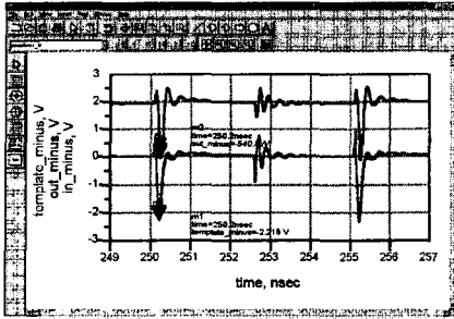
그림 11 (-) 펄스 복조기의 입출력 파형
