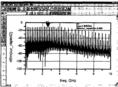
그림 8 (+) 펄스 변조기의 전력 스펙트럼
