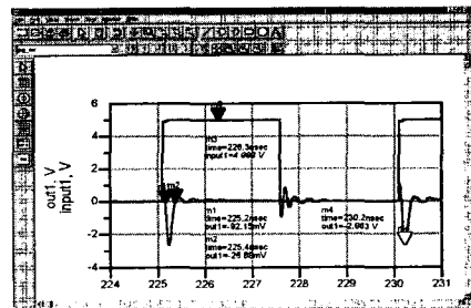
그림 5 (-) 펄스 변조기의 입출력 파형
