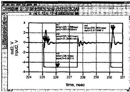
그림 6 (+) 펄스 변조기의 입출력 파형
