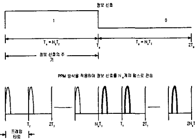
그림 1 PPM 방식에서 펄스의 구성
