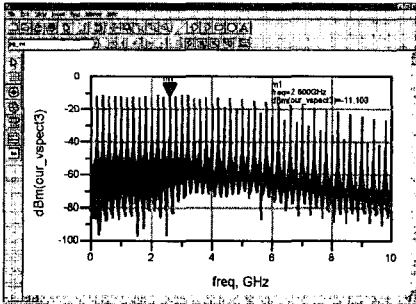
그림 7 (-) 펄스 변조기의 전력 스펙트럼
