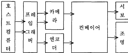
<그림 1> 시스템 구성도
