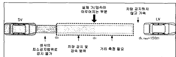
<그림 1> 시험 시 ACC 시스템의 제어 범위
