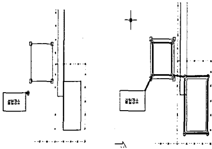
그림 1. 단일접지방식과 개선된 loop 접지방식
