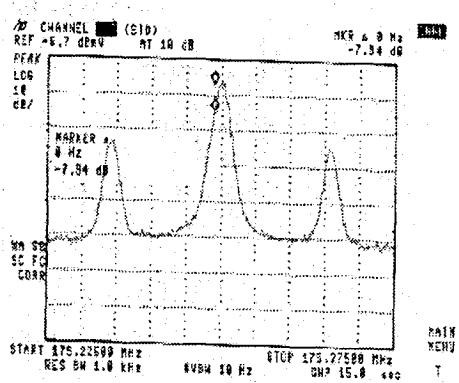
(a) 개선 전
