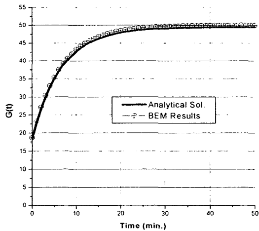
그림 2. 모서리 균열을 지닌 평판의 G(t)
