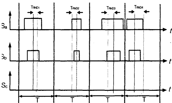
그림2 제안된 2상 RCD-PWM 각상의 펄스 Fig.2 Each phase pulse with the proposed two-phase RCD-PWM
