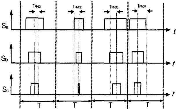
그림1 종전의 3상 RCD-PWM 각상의 펄스 Fig.1 Each phase pulse with conventional three-phase RCD-PWM
