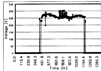
(d) Voltage waveforms
