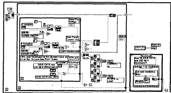
그림 2 태양전지 특성 측정을 위한 블록도 Fig. 2 Block diagram for cell characteristic
