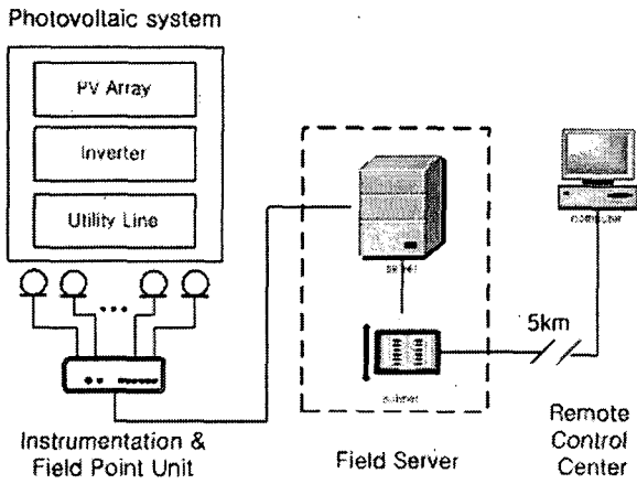
그림 1 시스템 구조 Fig. 1 Basic schematic of BIPV monitoring system
