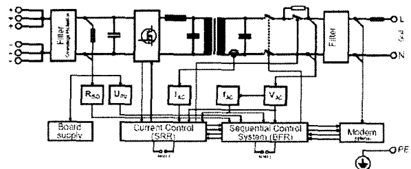
그림 3 인버터 블록 다이어그램 Fig. 3 Block diagram of Inverter
