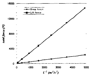
그림 5. 다양한 속도에 따른 차량의 Drag force와 Lift force
