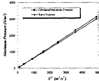
그림 4. 다양한 차량속도의 경우에 대한 최고압력과 이론 static pressure
