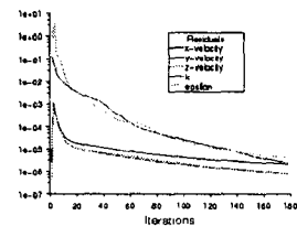
그림 3. Iteration 동안의 Residual의 변화 plot
