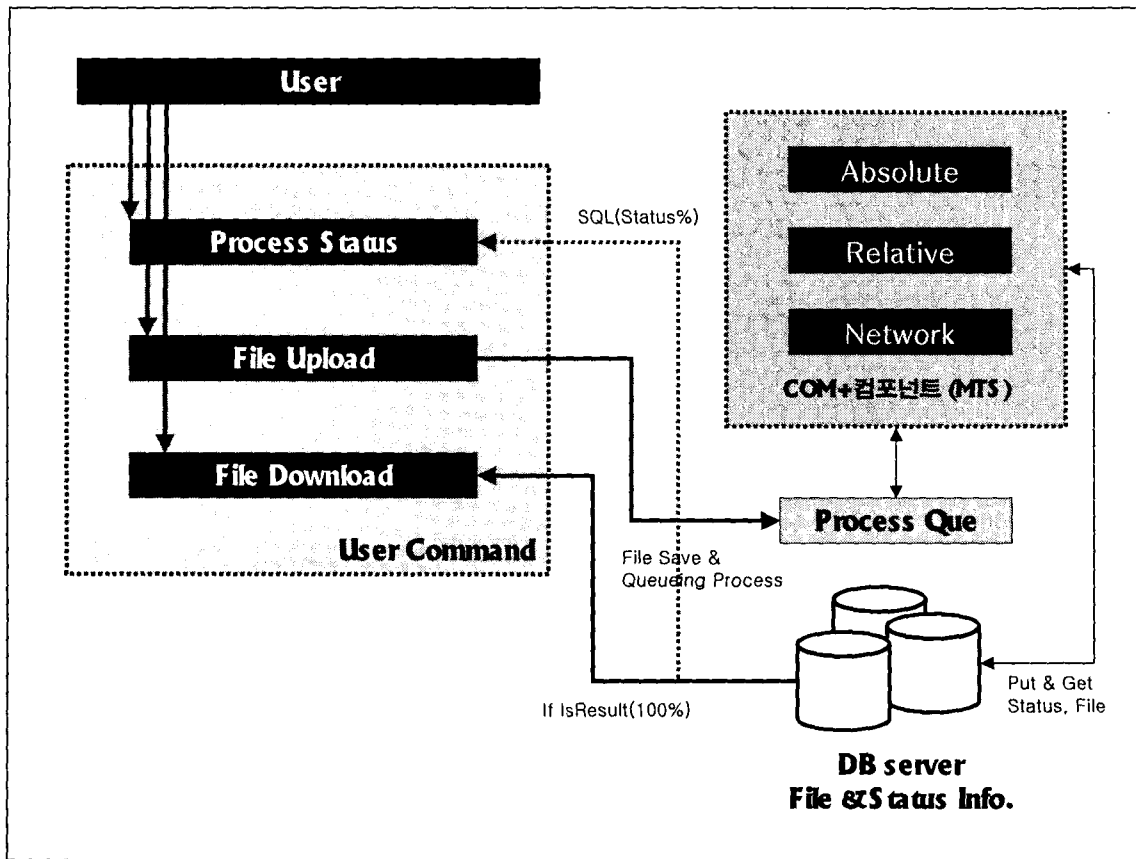
[그림 6] 웹기반 GPS 자료처리 시스템 개념도
