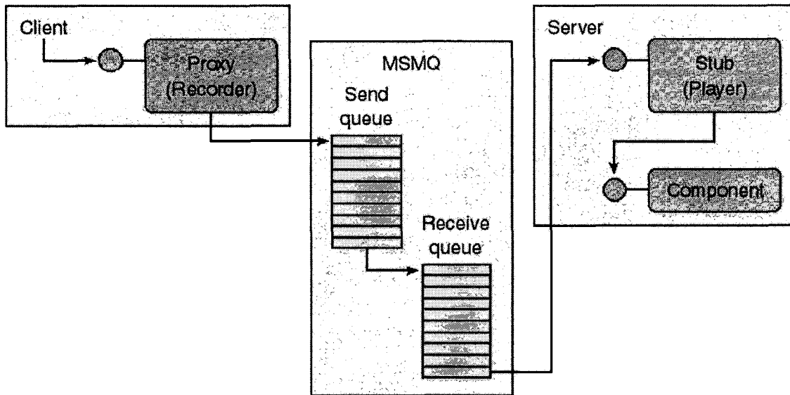
[그림 3] MTS & MSMQ 개념도(from Eddon and Eddon,1999)
