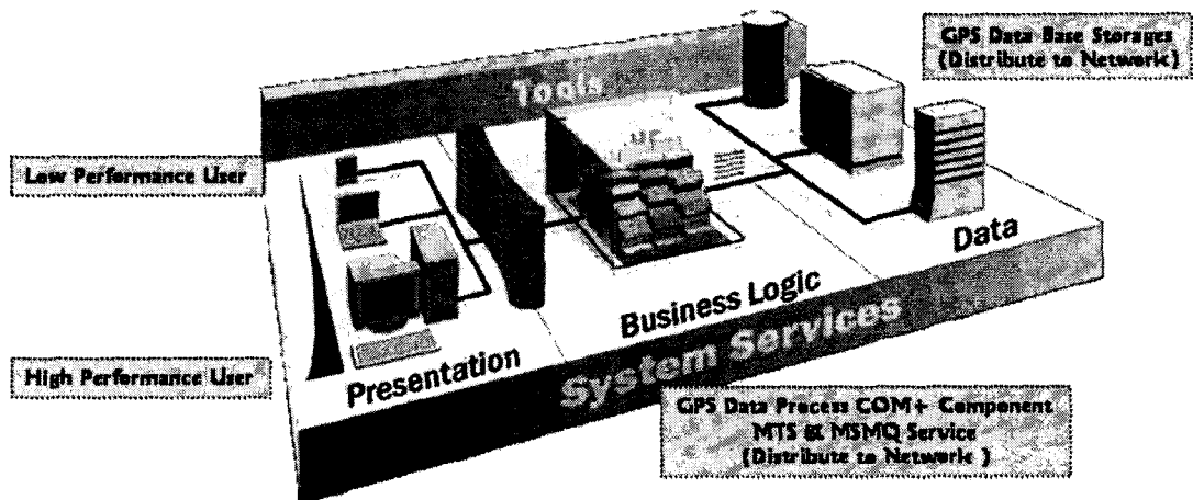
[그림 1] COM+ 시스템 개념도 (modified from Microsoft COM+ Knowledge Base Document)
