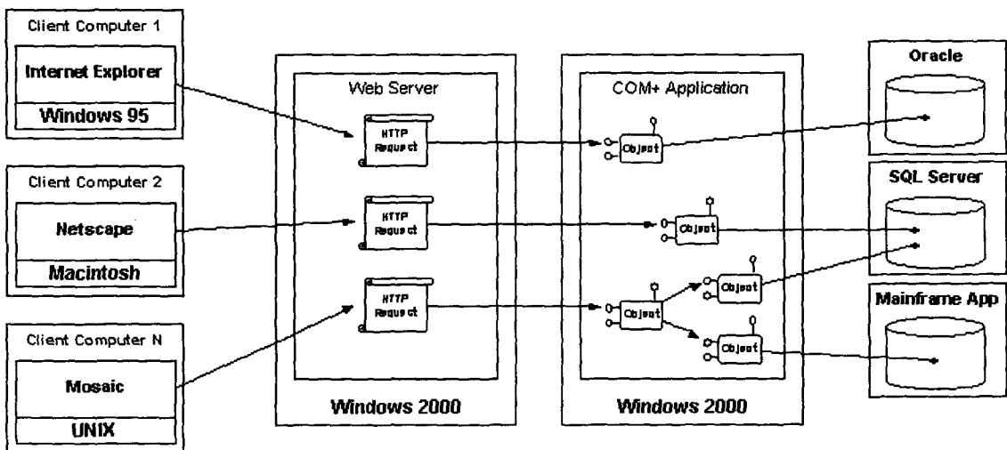
[그림 2] COM+ 기반 웹 시스템 다이어그램 (from Eddon and Eddon,1999)
