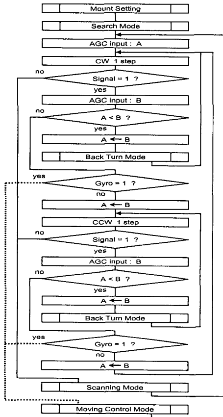
그림 6. 스텝트랙 알고리즘 Fig. 6 The algorithm on step track
