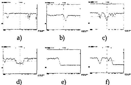
그림 12. 선박의 동요에 대한 보정 Fig. 12 Compensation for ship's moving
