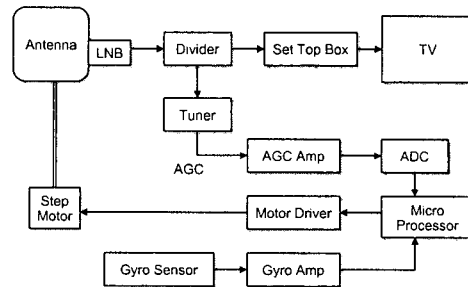
그림 2. 시스템의 구성도 Fig. 2 Block diagram of system
