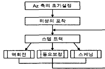
그림 5. 알고리즘의 구성 Fig. 5 Structure of algorithm
