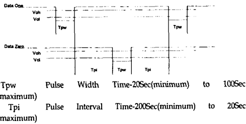
그림 6. 위겐트 신호 [4] Fig. 6 Wiegand Signal [4]
