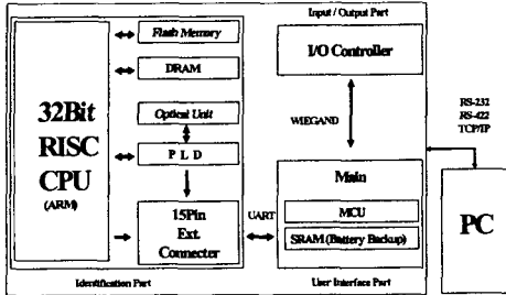
그림 1. 하드웨어 구조 블록도 Fig. 1 Hardware Block Diagram
