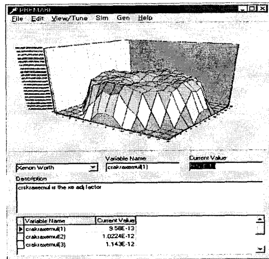
〈그림. 4〉 PRE-MARK 다이나믹 Viewer/Tuner
