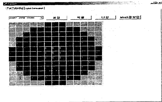
〈그림. 3〉 PREMARK 노심모델 입력자료 자동 생성틀-2
