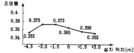
그림 7. 조명률의 변화 Fig. 7. Variation of utilization
