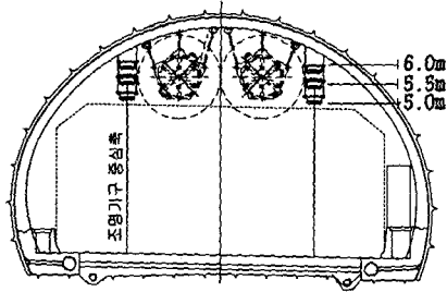
그림 11. 조명기구의 설치높이 Fig. 11. Mounting height of luminaire
