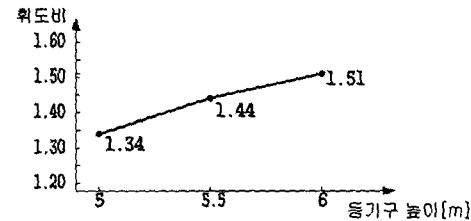
그림 13. 휘도비의 변화 Fig. 13. Variation of luminance
