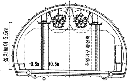
그림 14. 조명기구의 설치위치 Fig. 14. Mounting location of luminaire
