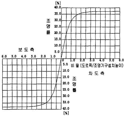
그림 1. 조명기구의 직사조명률 곡선 Fig. 1. Direct utilization factor curve of luminaire
