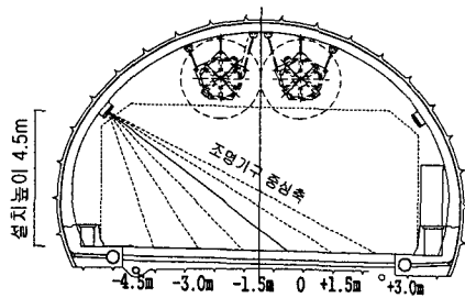
그림 6. 조명기구의 광축의 위치 Fig. 6. Location of luminaire axis
