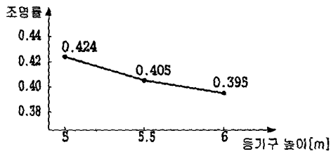
그림 12. 조명률의 변화 Fig. 12. Variation of utilization
