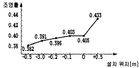
그림 15. 조명률의 변화 Fig. 15. Variation of utilization
