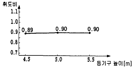
그림 5. 휘도비의 변화 Fig. 5. Variation of luminance
