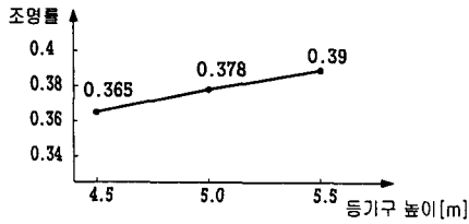
그림 4. 조명률의 변화 Fig. 4. Variation of utilization
