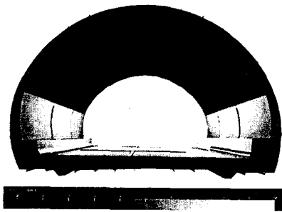
그림 9. 휘도 시뮬레이션 (단면도) Fig. 9. Luminance simulation (section)
