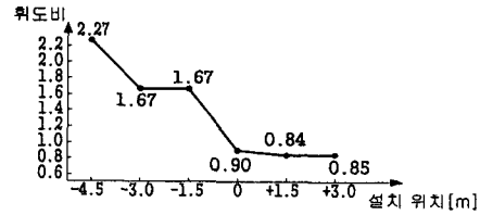
그림 8. 휘도비의 변화 Fig. 8. Variation of luminance
