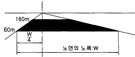
그림 2. 노면휘도의 측정 Fig. 2. Measurement of road surface luminance
