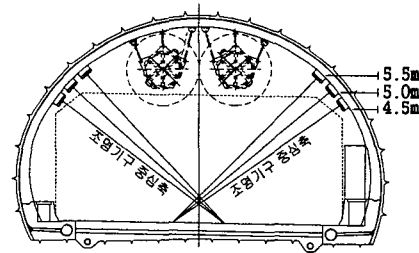
그림 3. 조명기구의 설치높이 Fig. 3. Mounting height of luminaire
