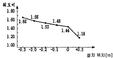
그림 16. 휘도비의 변화 Fig. 16. Variation of luminance
