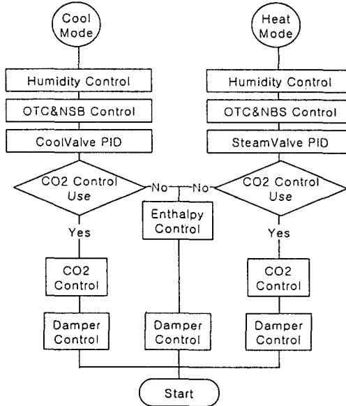
그림 2. AHU의 난방 및 냉방의 제어 로직 Fig. 2 Flow chart of Control logics of AHU heating and cooling
