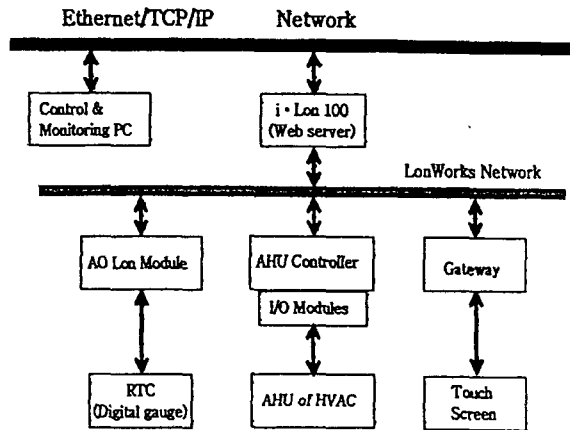
그림 5. 실험시스템 블록다이어그램
