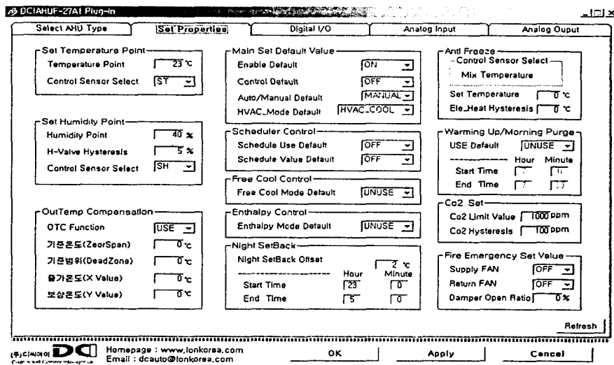
그림 4. AHU의 동작기능설정을 위한 Function Block Fig. 4 Function Block for setting controlling function of AHU
