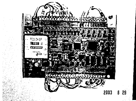
그림 1. 고성능 AHU 지능형제어 모듈 Fig. 1 Intelligent control module for AHU
