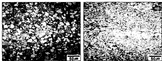
(c) equiaxed 950°C, 10^{-3} /s (d) widmanstätten 950°C, 10^{-3} /s
