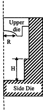
Fig. 2 Design Paramether(R, H) of open die
