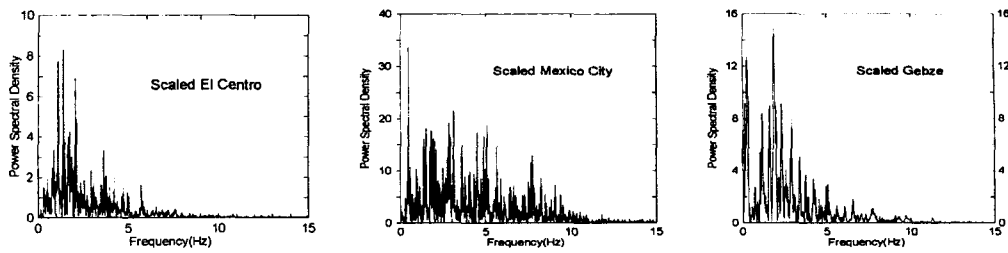
그림 4. 각 역사 지진의 Power Spectral Density
