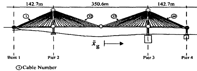
그림 2. 벤치마크 사장교모델(Dyke 등, 2003)
