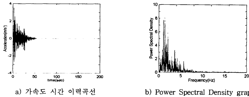
그림 3. 설계 지진 하중 (Scaled El Centro지진)
