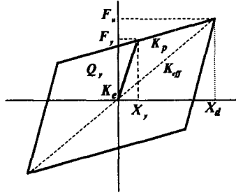
그림 1. 남고무 받침의 거동 및 설계 요소
